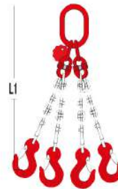
DÖRT BACAĞLI ZİNCİR SAPAN / FOUR LEGGED CHAIN SLING
